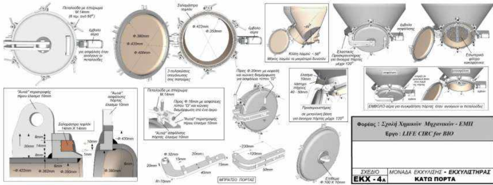
Σχήμα 5. Μονάδα εκχύλισης – Κάτω πόρτα εκχυλιστήρα
