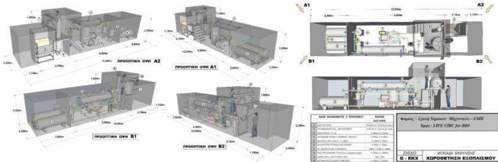
Σχήμα 1. Χωροθέτηση βασικού εξοπλισμού πρωτότυπης μονάδας εκχύλισης με ενσωματωμένο σύστημα για την ανάκτηση και ανακύκλωση διαλύτη
