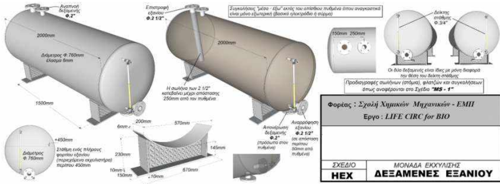
Σχήμα 11. Δεξαμενές εξανίου
