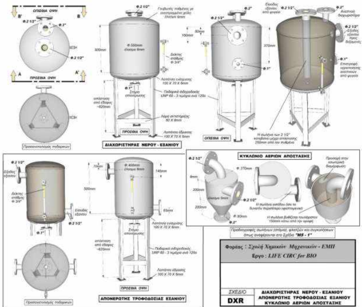
Σχήμα 12. Διαχωριστήρας νερού-εξανίου, απονερωτής τροφοδοσίας εξανίου και κυκλώνιο αερίων απόσταξης
