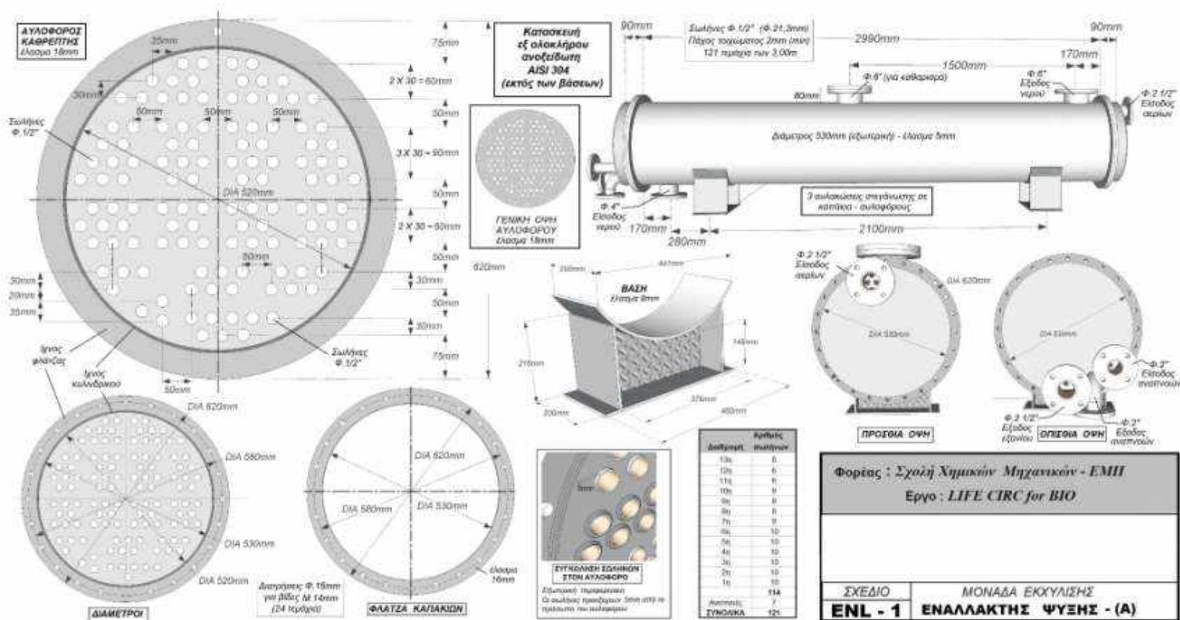
Σχήμα 9. Εναλλάκτης ψύξης
