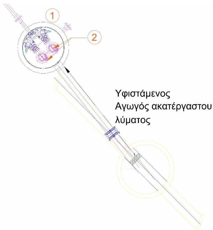
Σχήμα 1: Υφιστάμενος αγωγός με τον οποίο θα γίνει η σύνδεση της μονάδας (Αντλιοστάσιο και αγωγός ακατέργαστου λύματος) (Κάτοψη)
