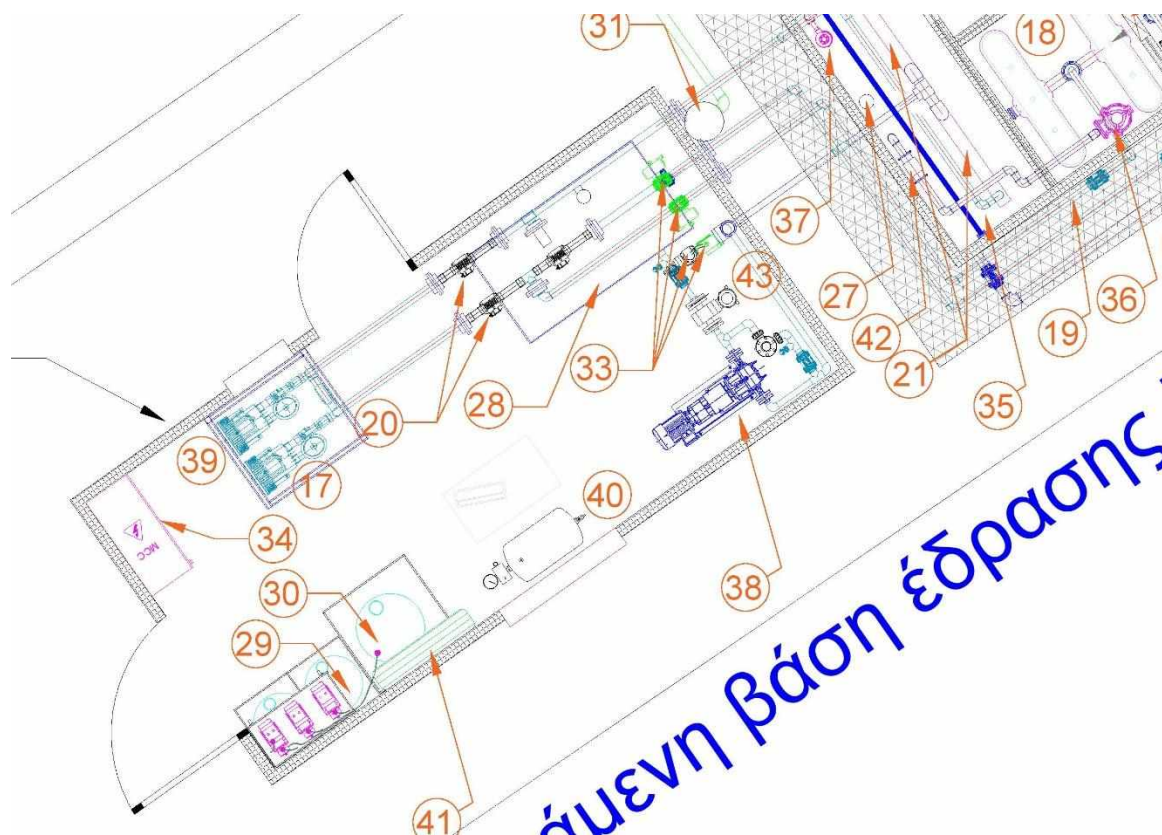
Σχήμα 6: Οικόσικος Ηλεκτρομηχανολογικού εξοπλισμού (Container machine room, Κάτοψη)
